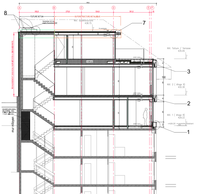
Coupe générale sur l'immeuble. Surélévation des deux étages et d'un attique.
